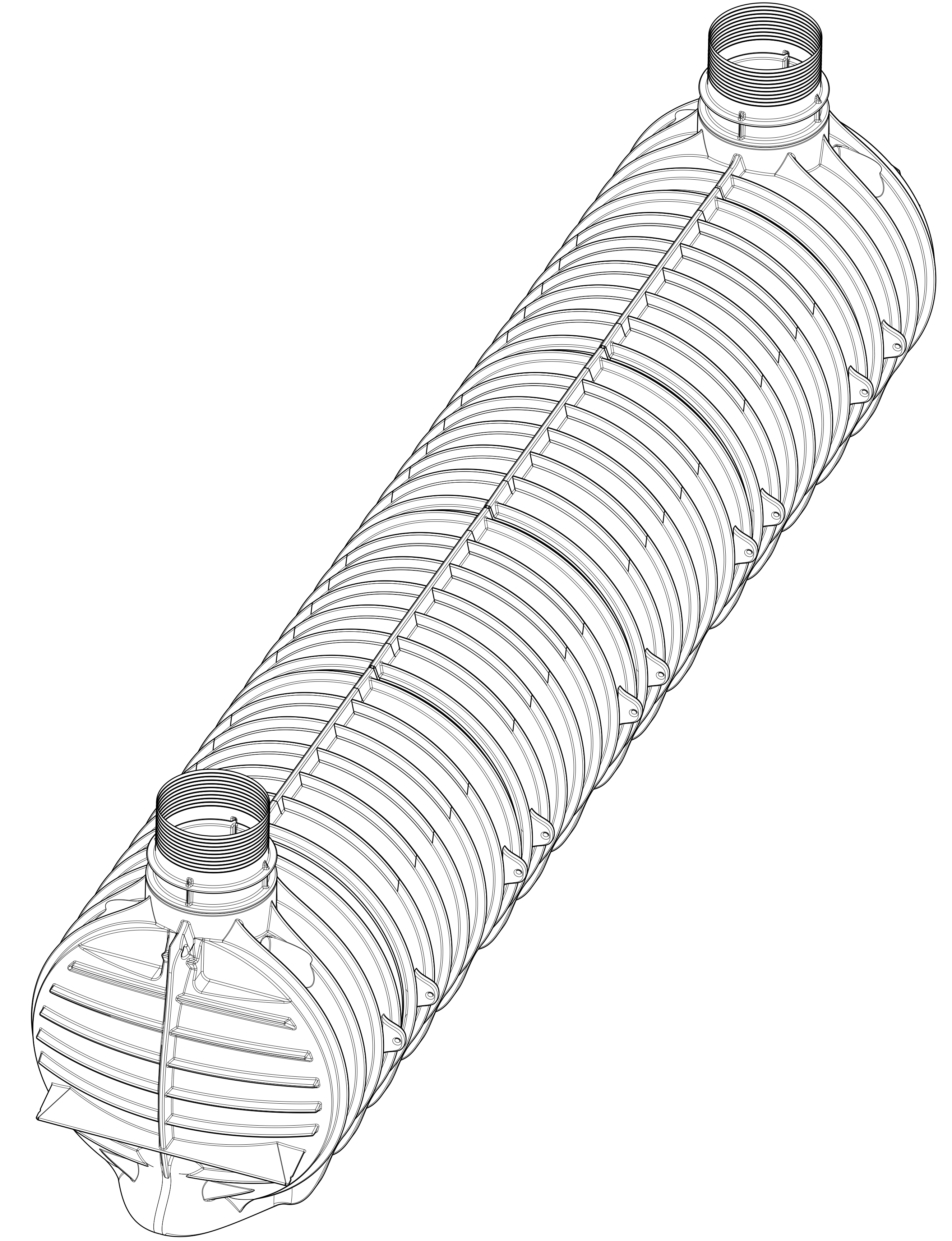
Isometric view Scale: 1:15
