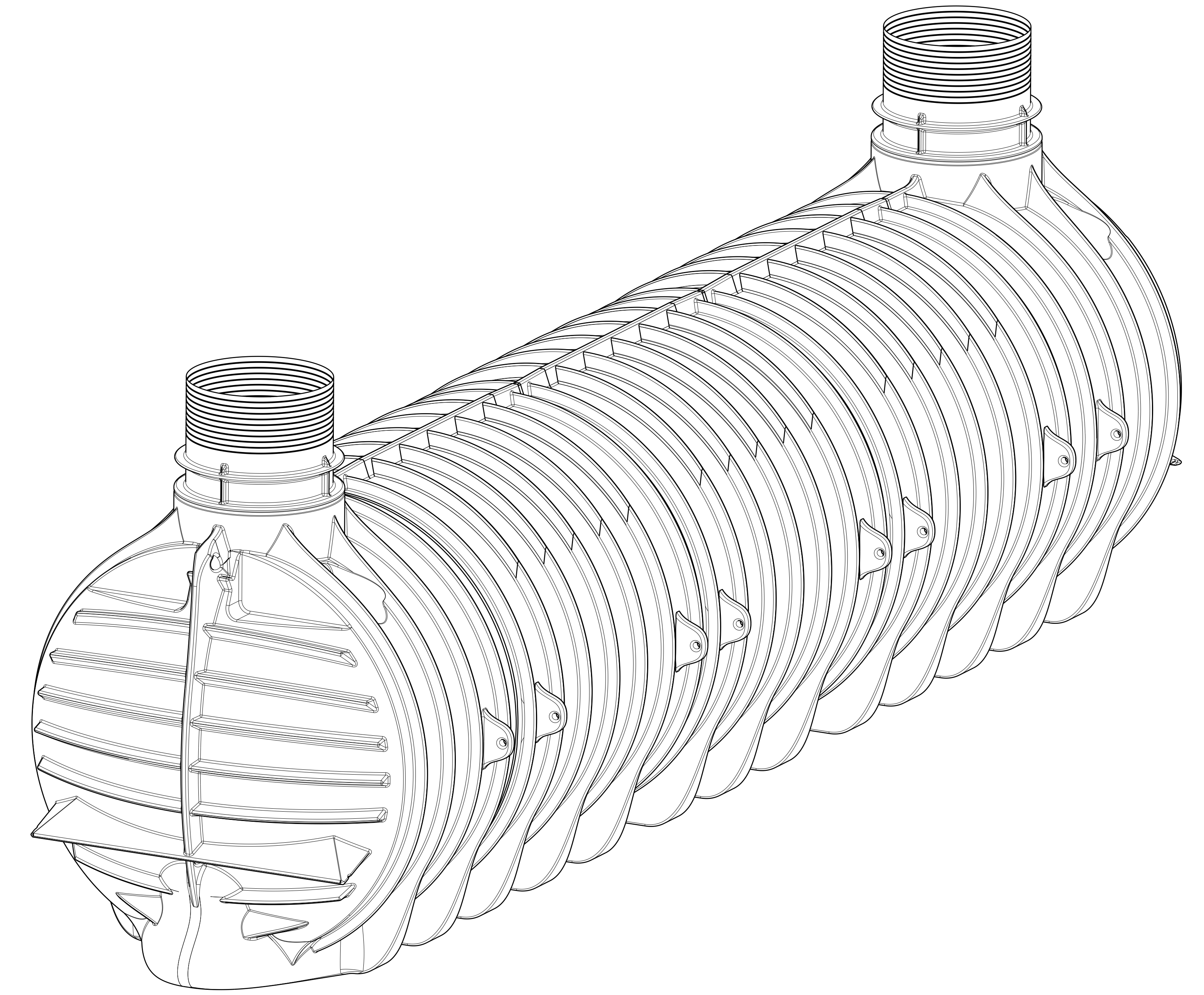
Isometric view Scale: 1:12
